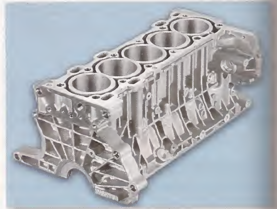
Camisa de motor policilíndrico
